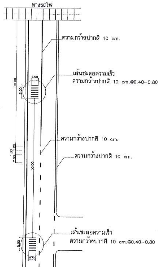
แบบงานตีเส้นจราจร
